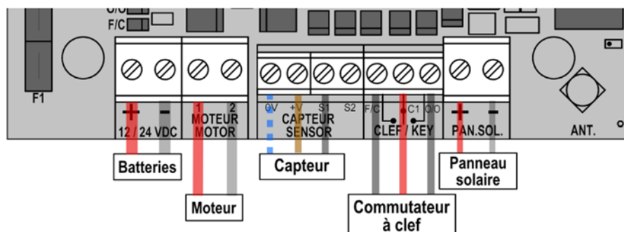
Schéma de câblage coffret AN35xx
